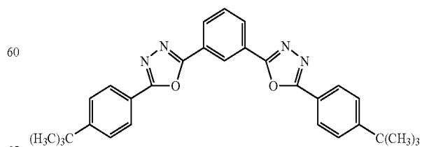
OXD-7
