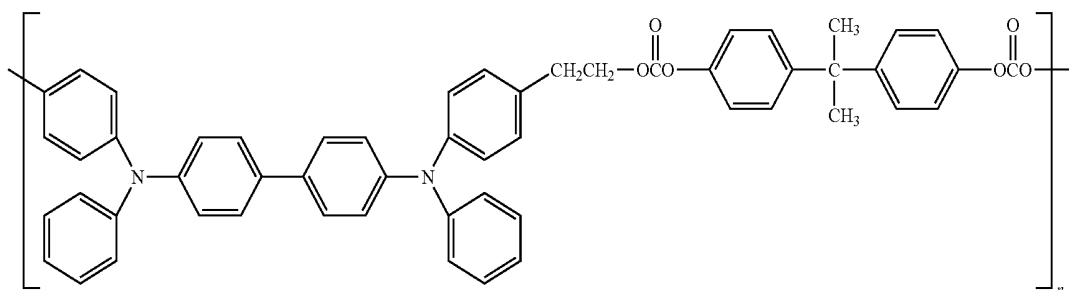
TPD-PCA
